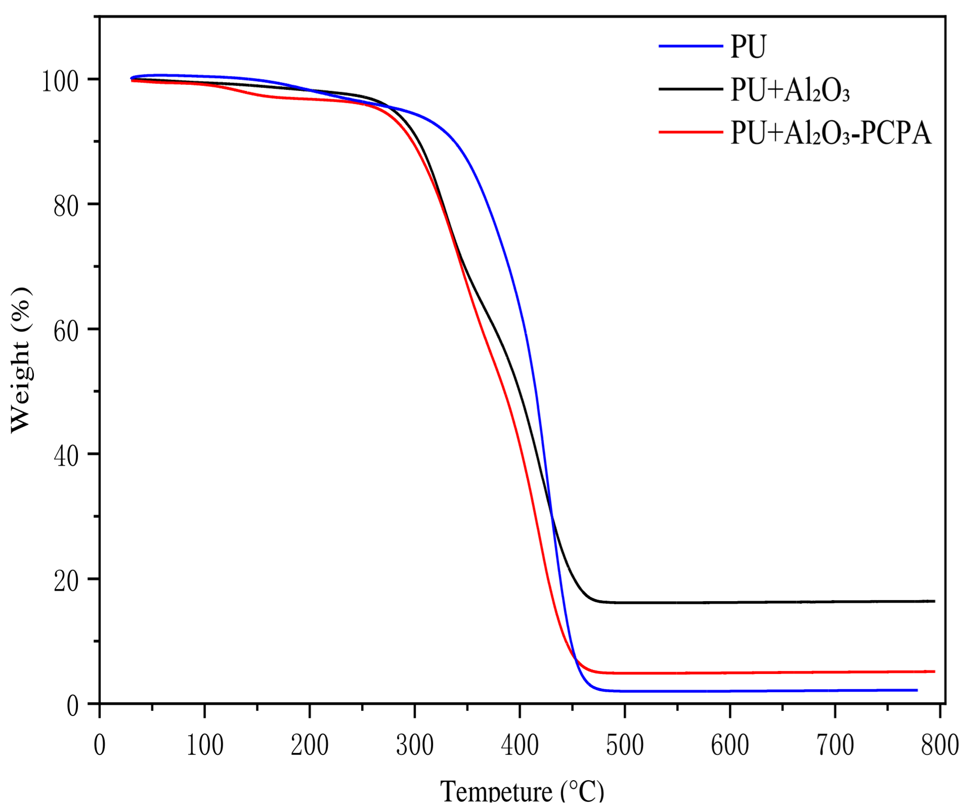
圖、一 (b) PU、PU+ Al 2 O 3 、PU+ Al 2 O 3 -PCPA 的 TGA 曲線
